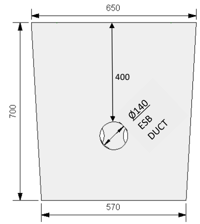
END ELEVATION
